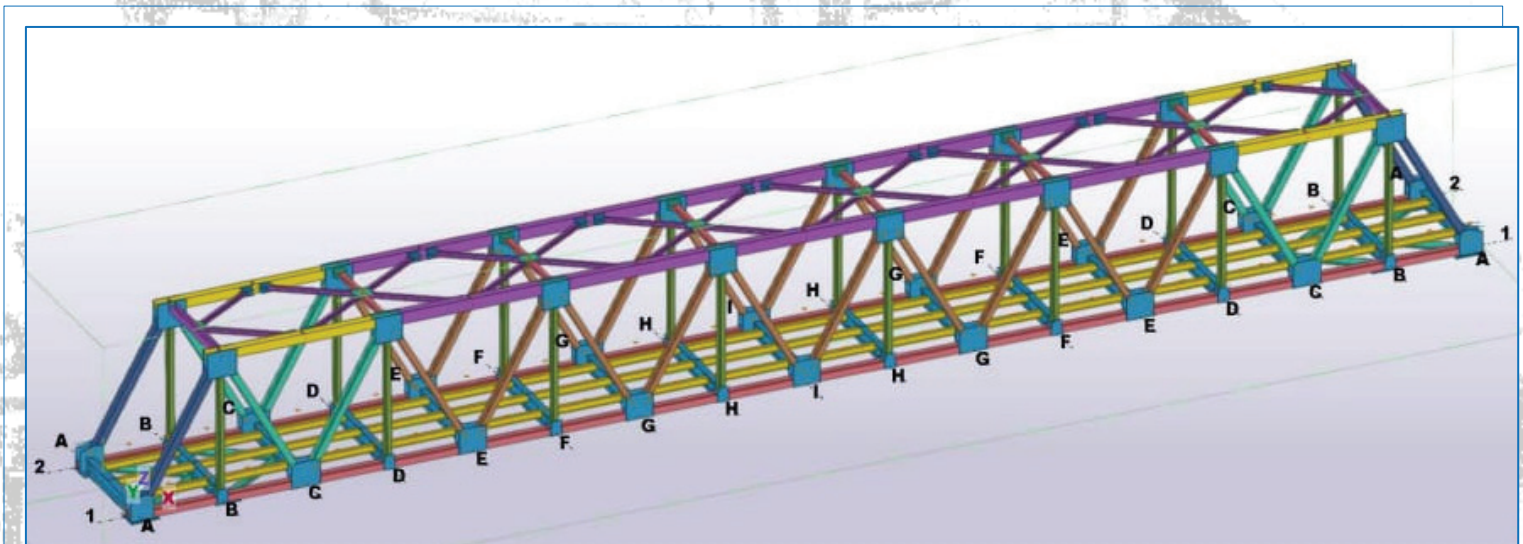
Diseño de Ingeniería del Puente Ramadillas 2021
